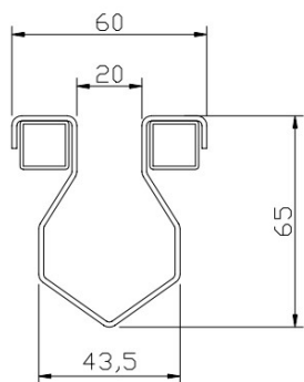
przekrój standardowy
