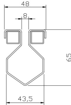
Querschnitt speziell für Schwimmbäder (Barfußbereich)
