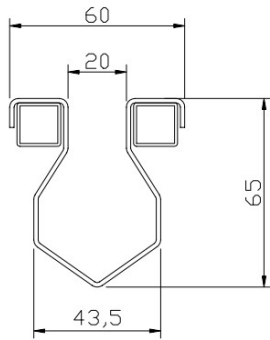
Standardquerschnitt
