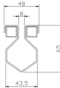
Querschnitt speziell für Schwimmbäder (Barfußbereich)
