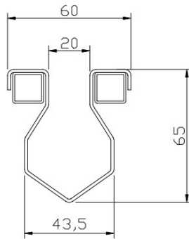
Standardquerschnitt
